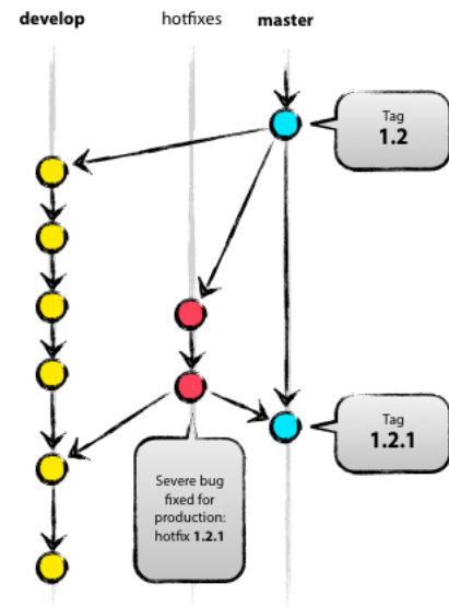
Рис. 4.6: Ветви исправлений (hotfix branches)
